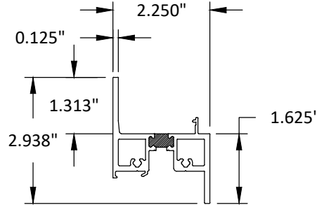
5 MULLION 6063-T5
