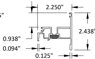
4 VENT 6063-T5
