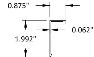
64 ANCHOR CLIP 6063-T5
