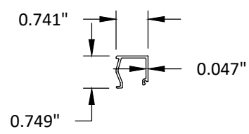
41 SMI GLASS STOP 6063-T5
