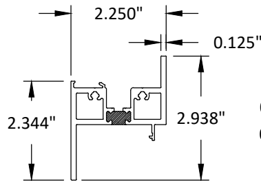
3 MULLION 6063-T5
