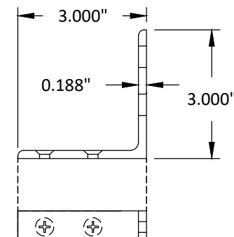
73 MULLION CLIP 6063-T5
