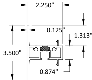
6 MULLION 6063-T5
