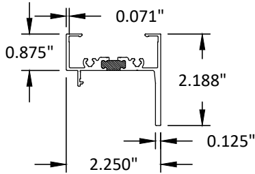
6 MULLION 6063-T5
