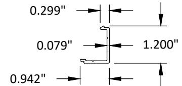
65 1 1/4" X 1" CLIP 6063-T5
