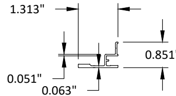
10 ADAPTOR 6063-T5
