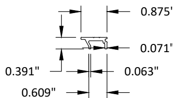
19 LOCK BAR BASE 6063-T5
